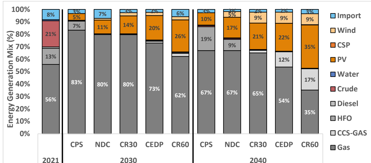
الشكل 14: مزيج إنتاج الطاقة بحسب نوع الوقود؛ 2021، 2030، 2040 (%)
