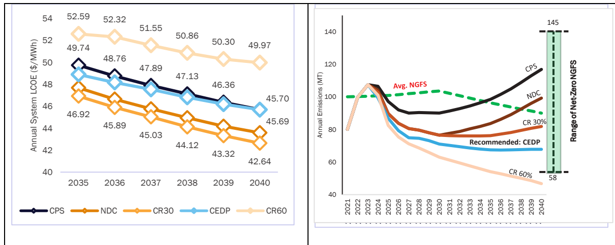
الشكل ES2: (أ) التكلفة السنوية للكهرباء وفق سيناريوهات مختلفة؛ (ب) الانبعاثات السنوية لقطاع الطاقة وفق سيناريوهات الكهرباء المختلفة
