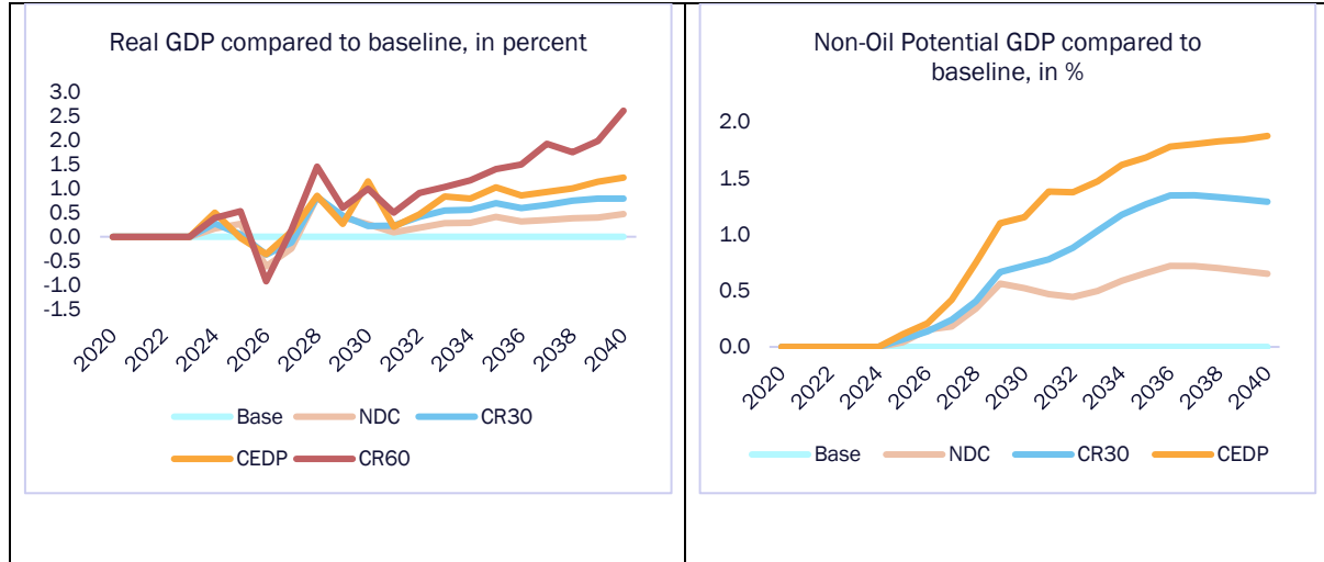
الشكل 19: (أ) مسارات تخفيض انبعاثات الكربون داعمة للنمو، (ب) وتزيد من إمكانات الناتج المحلي الإجمالي غير النفطي للبلد
