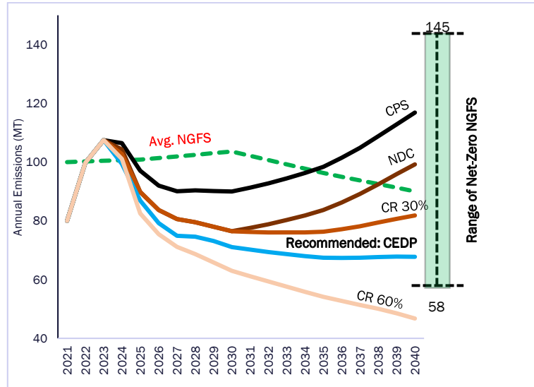
الشكل 15: الانبعاثات السنوية لقطاع الطاقة بحسب السيناريو
