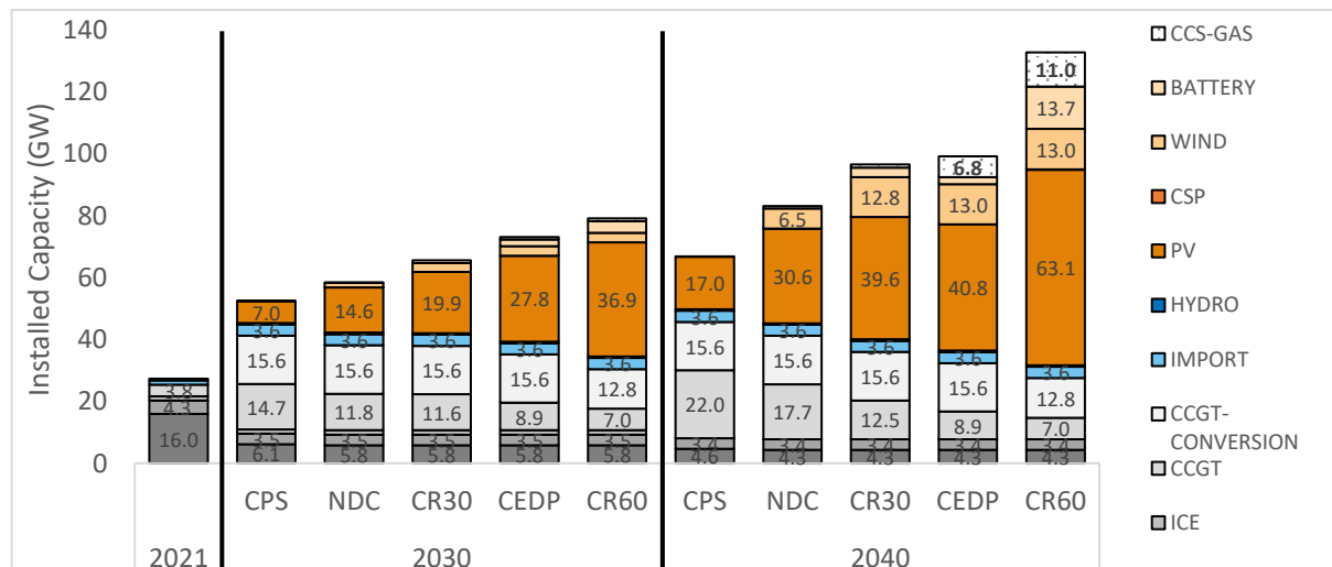
الشكل 13: السعة المُركّبة بحسب السيناريو؛ 2021، 2030، 2040 (جيجاوات)
