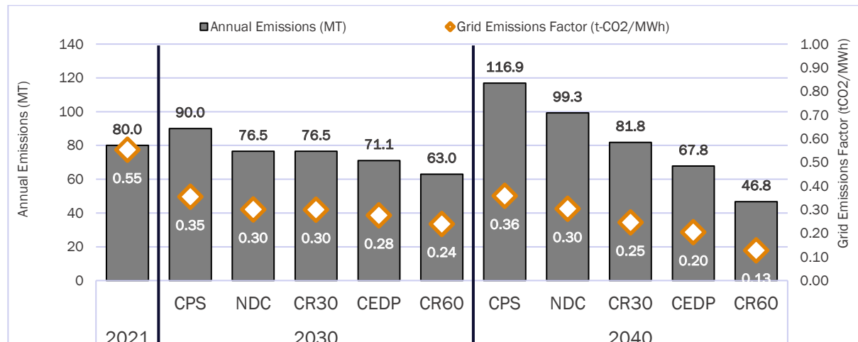
الشكل 16: الانبعاثات السنوية وكثافتها: 2021، 2030، 2040 (طن متري)
