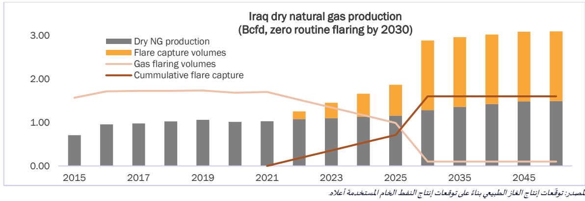
الشكل 10: توقّعات إنتاج الغاز الطبيعي الجاف في العراق (مليار متر مكعب في اليوم، مع التخلّص من حرق الغاز بحلول عام 2030)
